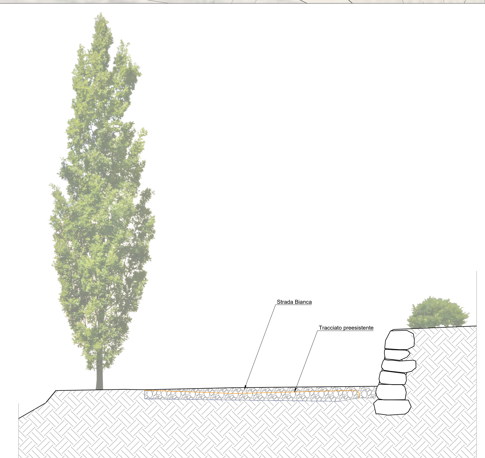
Sezione tipo F-F - scala 1:50
