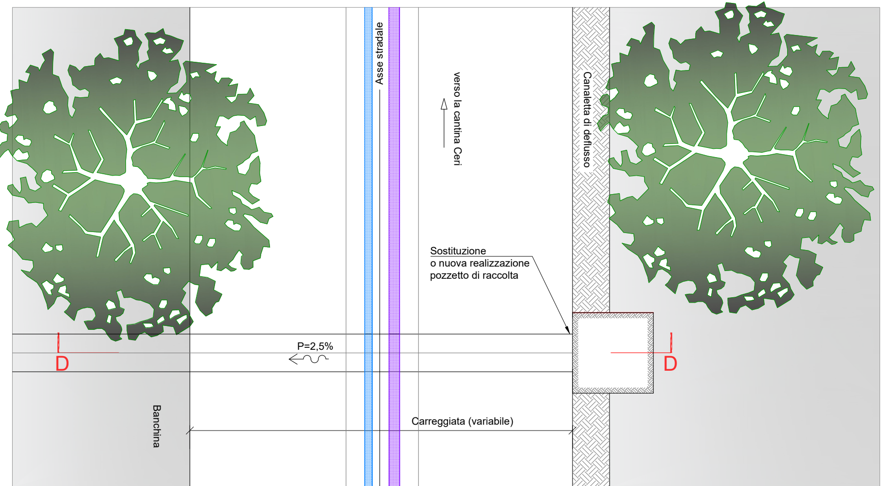
Pianta tipo - canaletta e pozzetto di raccolta acque_scala 1:50
