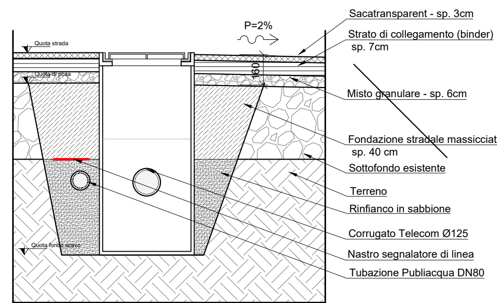
Dettaglio tipologico pozzetto Telecom 40 x 40 - scala 1:20
