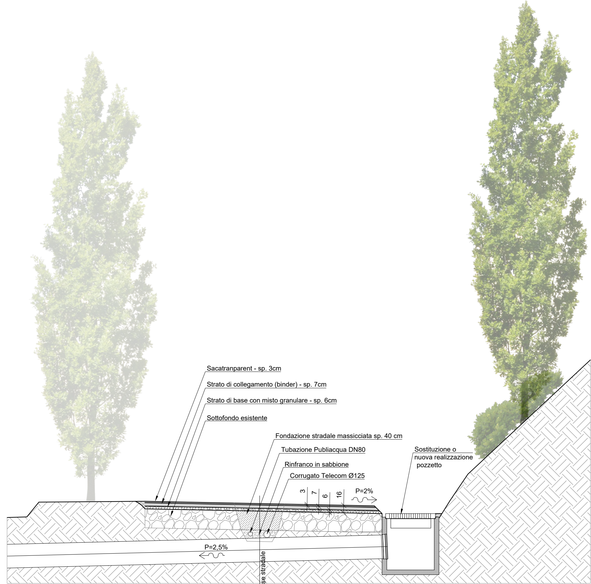
Sezione tipo D-D - scala 1:50
