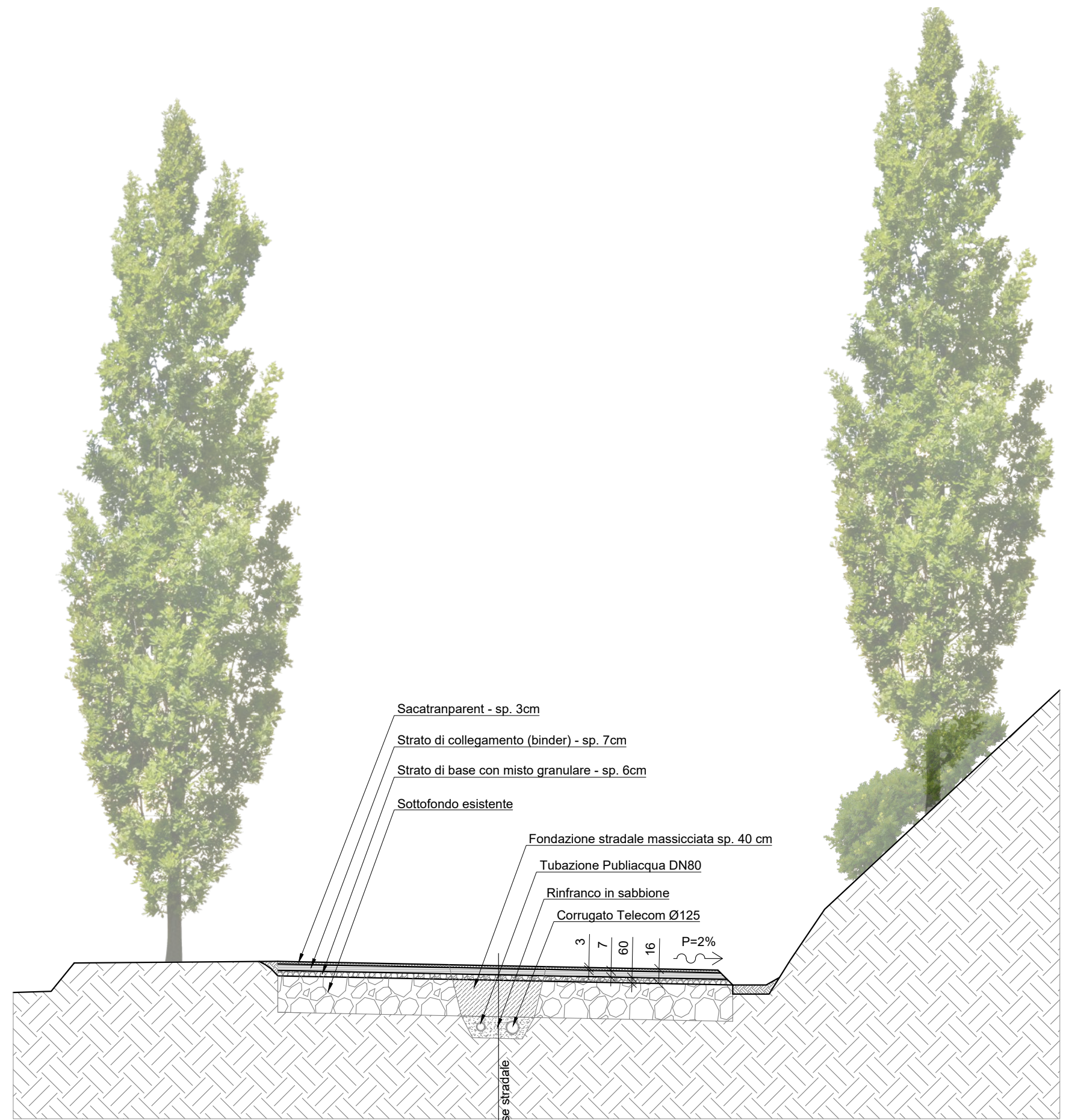
Sezione tipo E-E - scala 1:50
