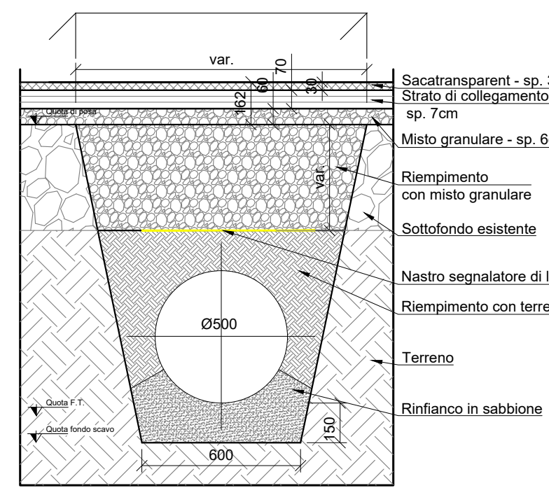
Dettaglio tipologico scavi scarico acque - scala 1:20
