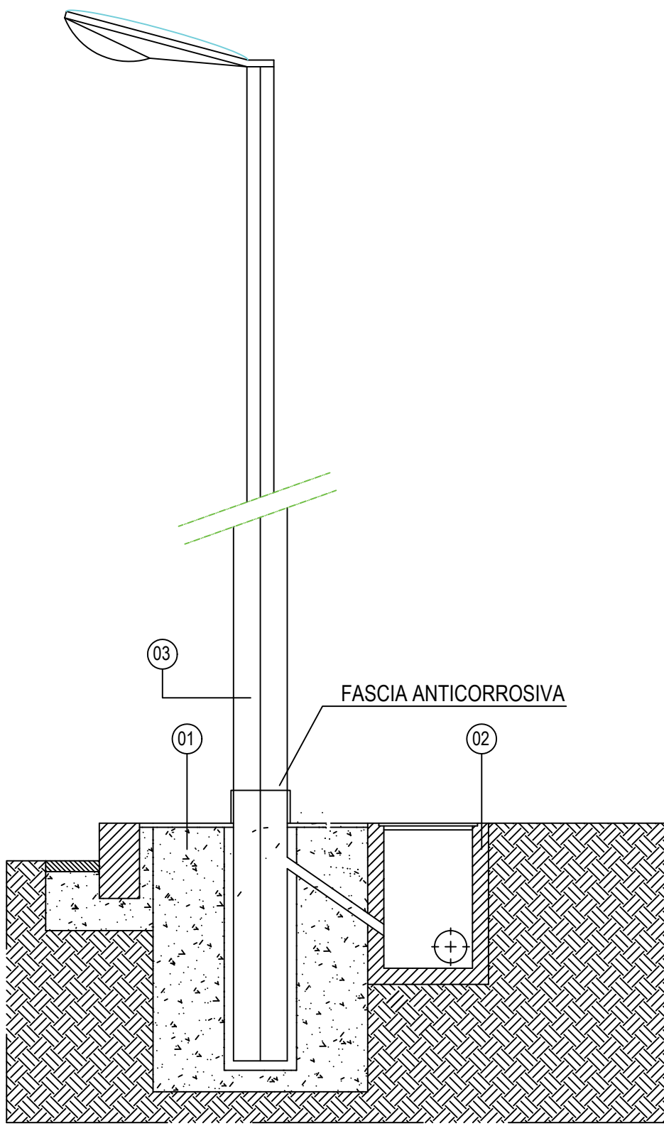
Part. - Basamento palo
